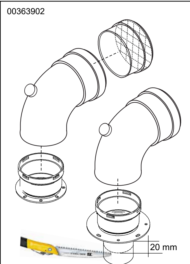
Nota: Tagliare alla quota indicata Installazioni Tipo B22 per esterno
