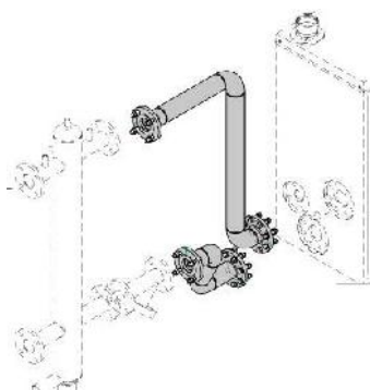
Levostranné připojení sběrače
