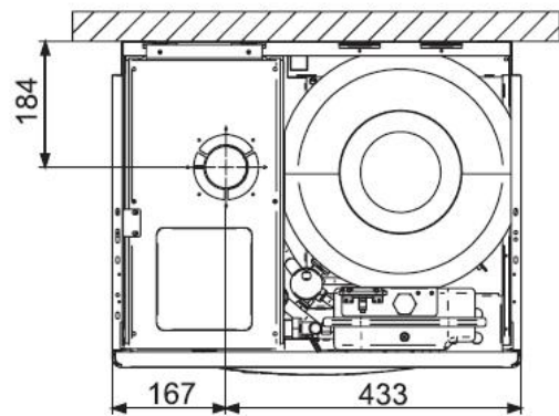
Pohled zespoda
